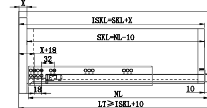
GAVETA EMBUTIDA:
