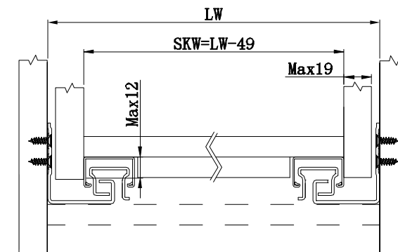
GAVETA EMBUTIDA:
