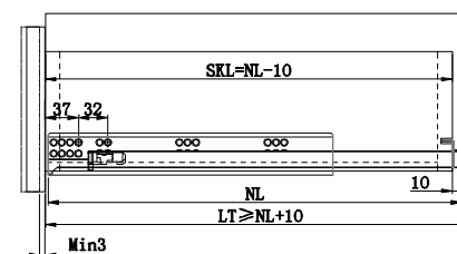
GAVETA SOBREPOR:
